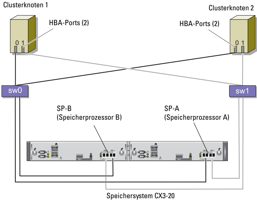
Abbildung 1-2. Dell|EMC SAN-verbundenen Fibre-Channel-Cluster verkabeln
