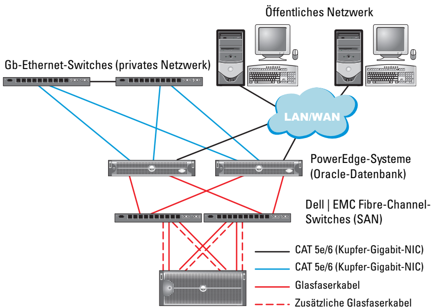
Abbildung 1-1. Hardwareverbindungen für einen SAN-Attached Fibre-Channel-Cluster
