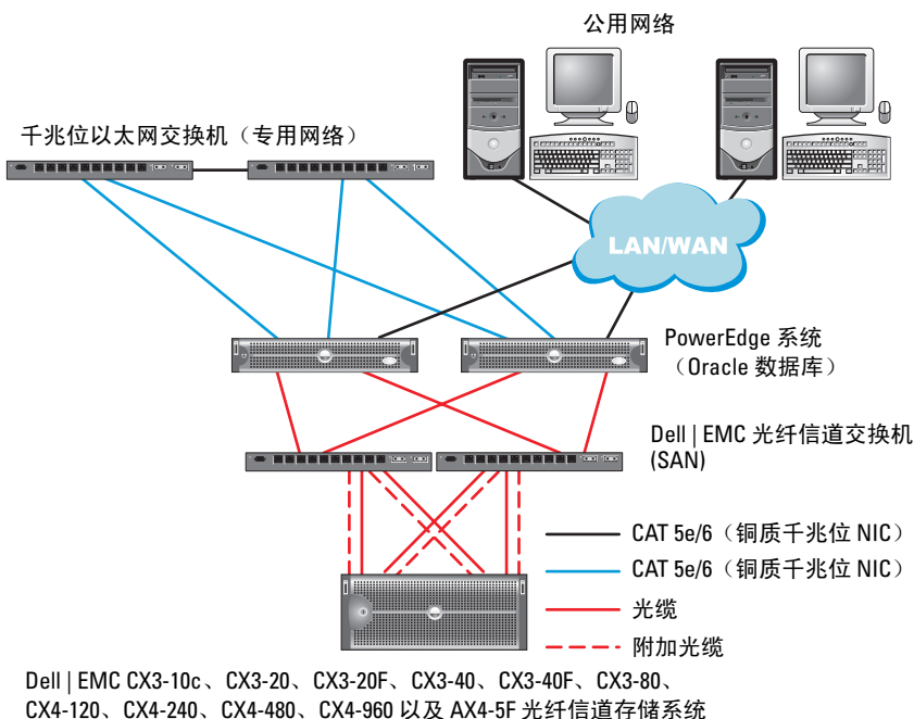
图 1-1. SAN 连接的光纤信道群集的硬件连接
