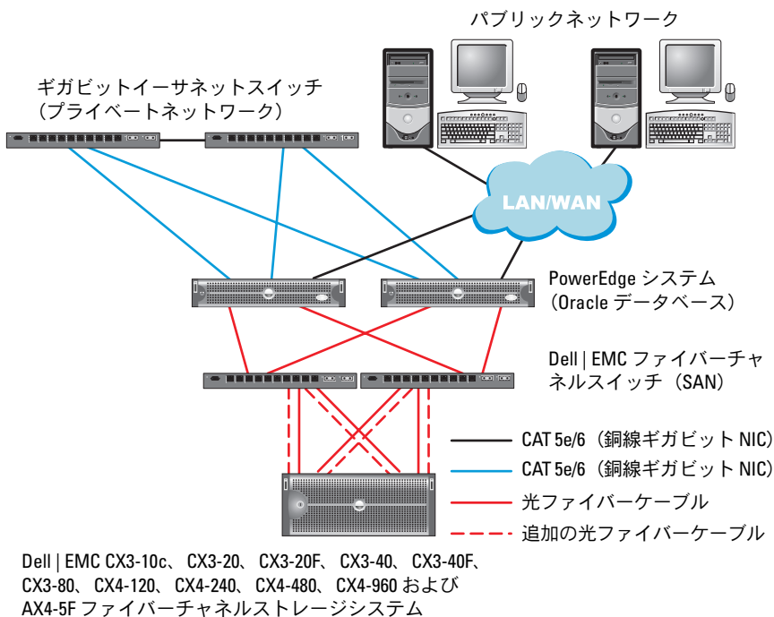
図 1-1 SAN 接続のファイバーチャネルクラスタ用のハードウェア接続
