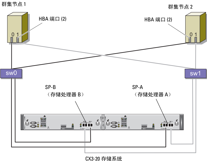
图 1-2. 在 Dell|EMC SAN 连接光纤信道群集中布线
